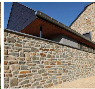
Rohemauerwerk Bruchsteine
